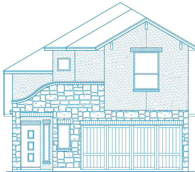
Elevation B
